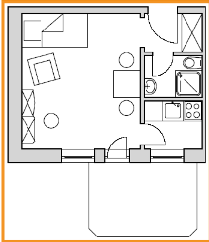
Appartement für 1 - 2 Personen im Erdgeschoss. Grundrissfläche: ca. 23 m 2
